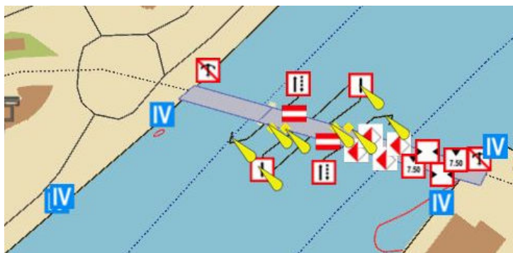
Rysunek 7. Dane przetworzone zgodnie z algorytmem dla skali 1:2000, przedstawione w geokompozycji składowej 1:5000 (obraz powiększony, aby ułatwić ocenę)
