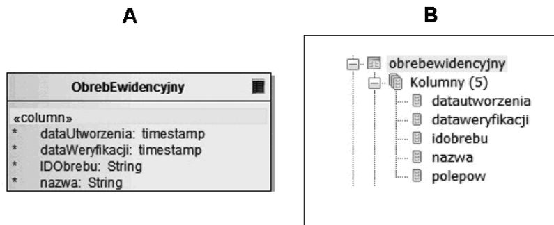
Rys. 10.7. A – Atrybuty ze stereotypem «column» w klasie UML.
