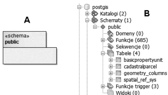
Rys. 10.4. A – Pakiet ze stereotypem «schema». B – Reprezentacja schematu w oknie elementów modelu SZBD PostgreSQL/PostGIS.
