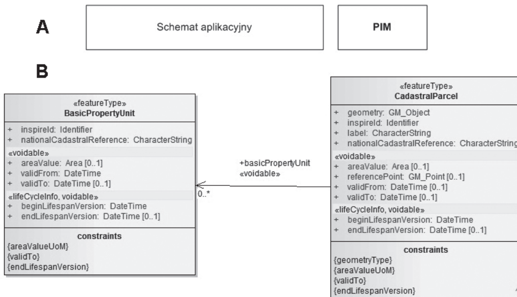
Rys. 10.11. A – Poglądowe przedstawienie kroku 1. B – Fragment schematu aplikacyjnego INSPIRE dotyczącego tematu działki ewidencyjne (TWG-CP, 2010).
