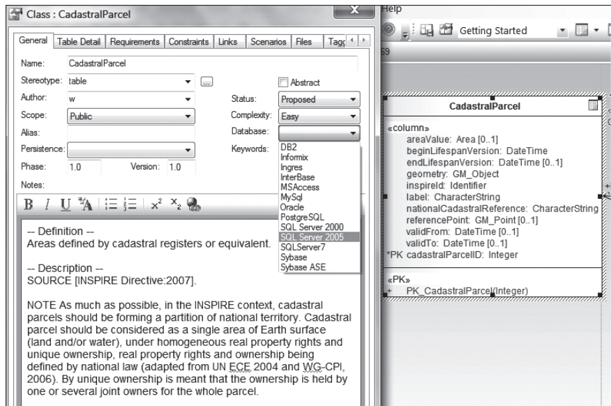
Rys. 10.14. Wybór docelowej bazy danych – lista SZBD dostępna w programie Enterprise Architect w polu o nazwie Database.
