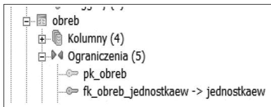
Rys. 10.10. Oznaczenie klucza obcego w oknie elementów modelu SZBD PostgreSQL/PostGIS.
