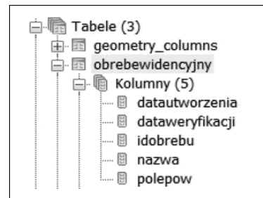
Rys. 10.6. Reprezentacja tabeli w oknie elementów modelu SZBD PostgreSQL/PostGIS.
