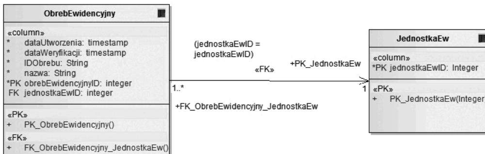
Rys. 10.9. Oznaczenie klucza obcego w klasie UML.
