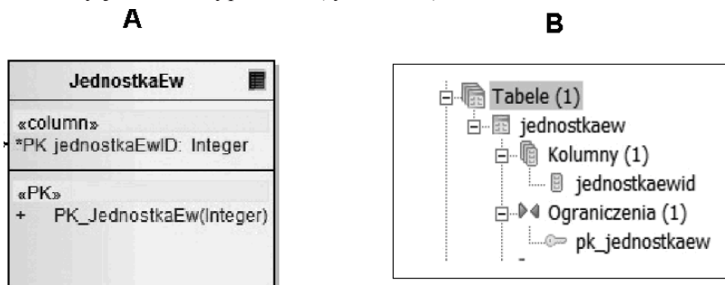
Rys. 10.8. A – Oznaczenie klucza głównego w klasie UML. B – Oznaczenie klucza głównego w oknie elementów modelu SZBD PostgreSQL/PostGIS.
