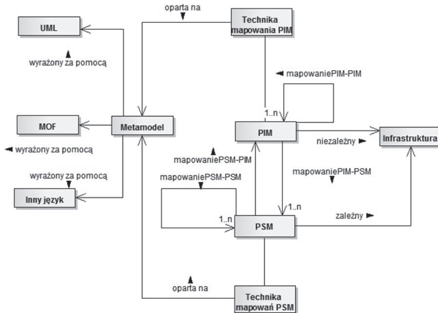
Rys. 10.2. Diagram klas przedstawiający metodykę MDA. Źródło: opracowanie własne na podstawie przewodnika MDA (OMG, 2003).
