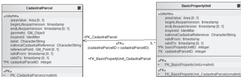
Rys.10.13. Wynik transformacji do DDL – model PSM.
