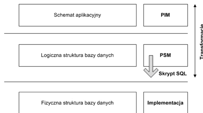
Rys. 10.1. Transformacja schematu aplikacyjnego do struktury bazy danych w kategoriach pojęć MDA.
