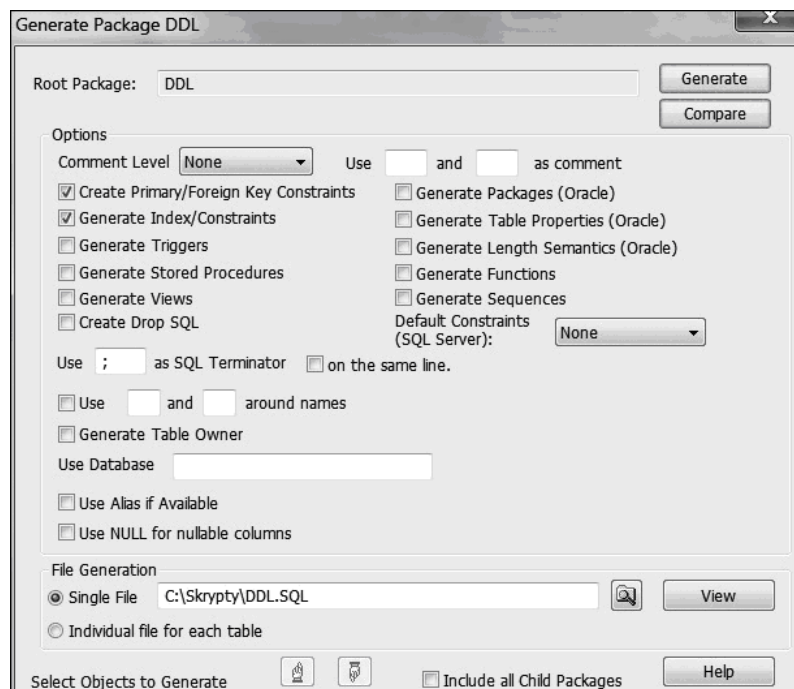
Rys. 10.15. Okno ustawień procesu generowania skryptu DDL.
