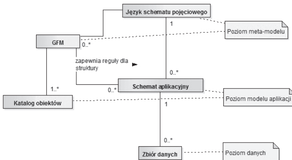
Rys. 5.2. Związek między Ogólnym Modelem Obiektów (GFM), schematem aplikacyjnym i zbiorem danych (ISO/TC 211, 2002a).
