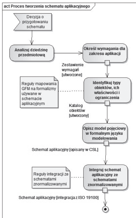
Rys. 5.3. Proces budowy schematu aplikacyjnego.
