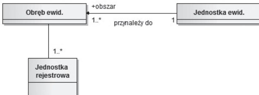
Rys. 5.4. Fragment schematu aplikacyjnego bazy danych ewidencyjnych.
