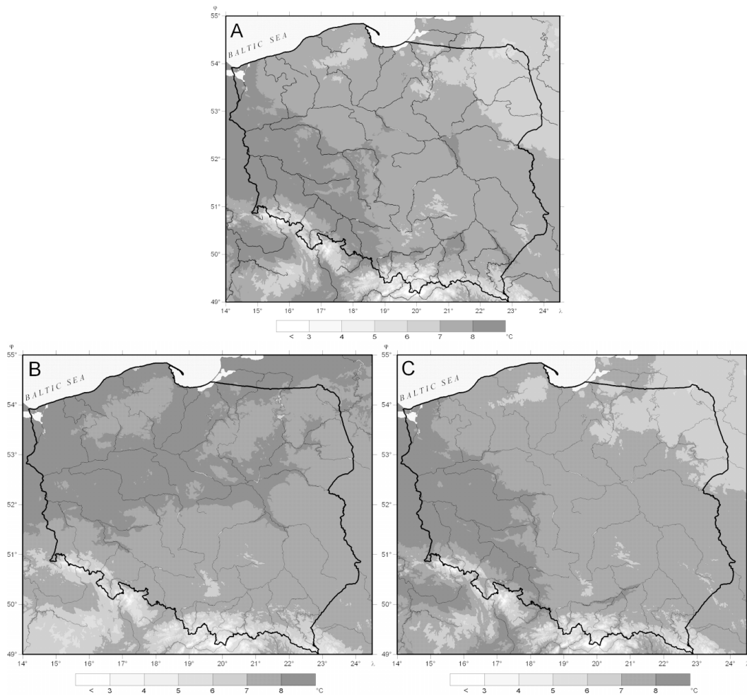
Rys. 1. Średnia roczna temperatura powietrza w Polsce wg 3 różnych metod spacjiacji: A – kriging resztowy, B – regresja prosta, C – regresja wielokrotna
