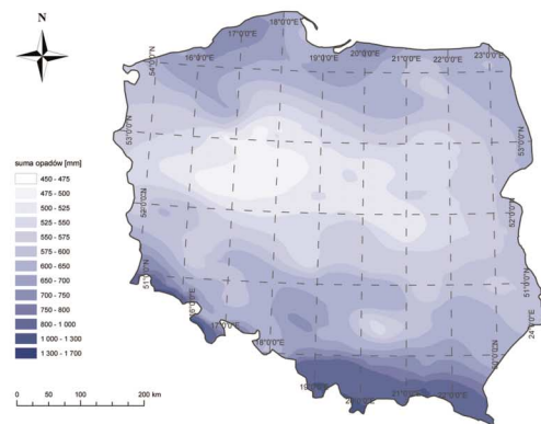
metoda interpolacji: kriging prosty
