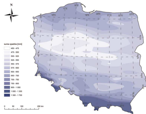
metoda interpolacji: cokriging zwykły
