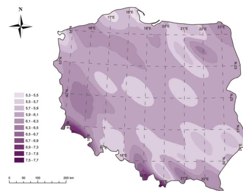
Rys. 3. Średnie roczne oraz miesięczne (styczeń, luty, czerwiec) zachmurzenie ogólne (oktany)
