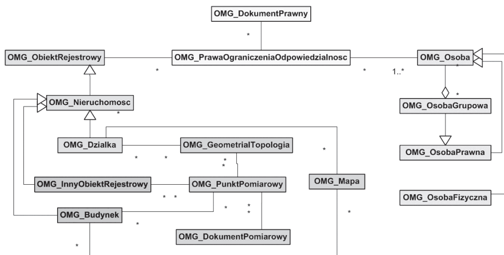
Rys. 8.1. Szkic Ogólnego Modelu Geodezyjnego
