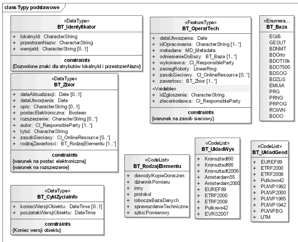
Rys. 8.4. Model „Typy Podstawowe”.
