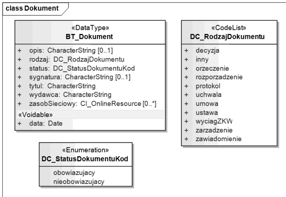
Rys. 8.3. Model „Dokument”.
