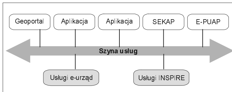
Rys. 1. Architektura węzła IUIP. Objaśnienia: SEKAP – System Komunikacji Administracji Publicznej w województwie śląskim, ePUAP – Elektroniczna Platforma Usług Administracji Publicznej
